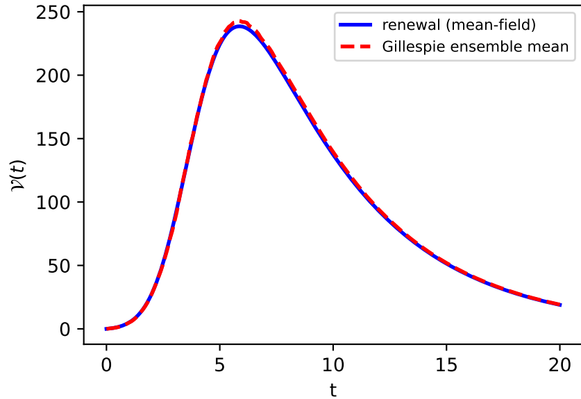
Free virus (mu_pos)
